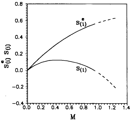
Рис.1 Зависимость энтропии на внешней s_i^e и внутренней s_i сторонах кнудсеновского слоя от числа Маха в модели [3].
